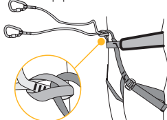
Installing webbing to harness. Připojení k sedacímu úvazku.
